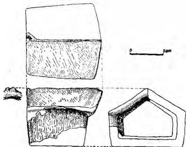
Fig. IVc.29. Machet\ de cuptor de la Radovanu, dup\ Com[a
