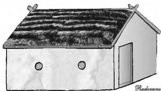
Fig. IVc.22a. Radovanu, locuință (reconstituire E. Com[ă)
