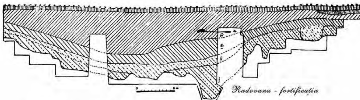
Fig. 41 Profilul secțiunii (executată în partea de vest a complexului) prin șanțul de apărare: I = nivelul de săpare a șanțului; II-III = niveluri de umplere și IV = corespunzător nivelului 1 din așezare și mai ales solului depus în milenii următoare, inclusiv unele deranjamente feudale târzii.
