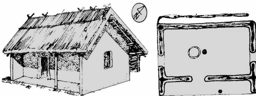
Fig. IVc.19. Locuin]e de la Petru Rareș [▲ [i Tangâru ▼, dup\ Hoin\rescu
