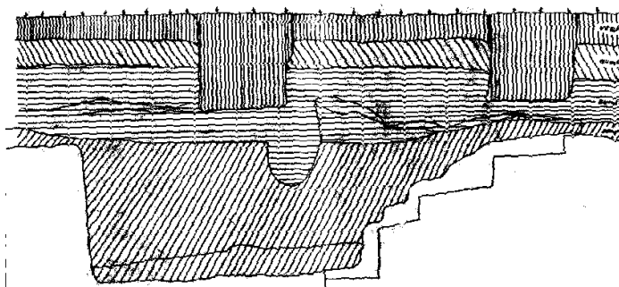
Fig. IVc.15. Bordei, Li[coteanca, după Harjuche
